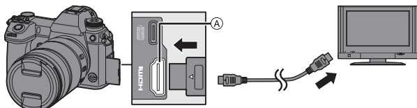
Ⓐ Konektor [HDMI] (Typu A)
